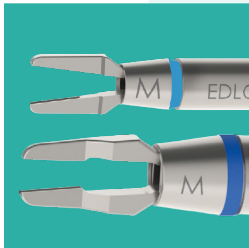
Aplicador de Clip SLS Médio (Azul) Ø6,5mm e Ø10mm 14-1495, 14-1493, 14-1496, 14-1494, 14-1489, 14-1487, 14-1490 e 14-1488
