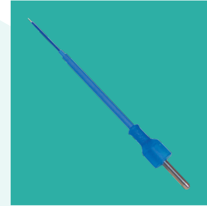
Eletrodo Agulha Microcirúrgica com Sleeve ™ de Segurança Isolada / Compr. Tot.: 10,16cm / Compr. Exp.: 9cm / Compr. Atv.: 3mm / Raio da Ponta: 0,06mm
