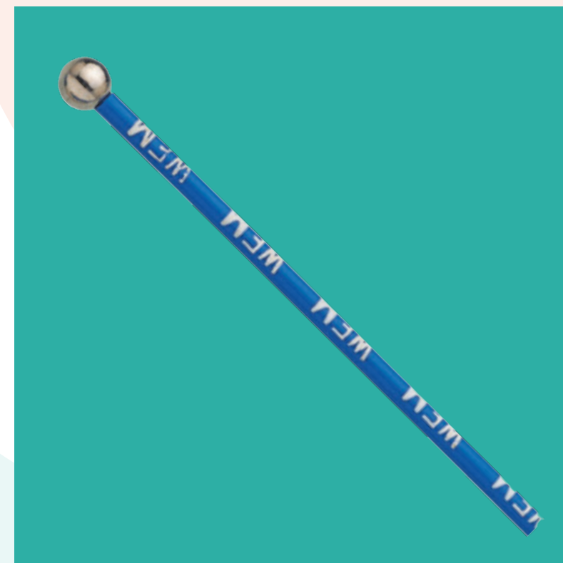
Eletrodo Médico 75mm Ponta Tipo Bola Ø 4,76mm (E-100)
