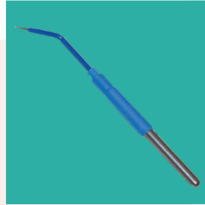
Eletrodo Agulha Microcirúrgica Isolada Comp. Tot.: 5,4cm / Comp. Exp.: 3cm / Comp. Atv.: 3 mm / Raio da Ponta: 0,06 mm / Ângulo de 45° / 1cm da Ponta
