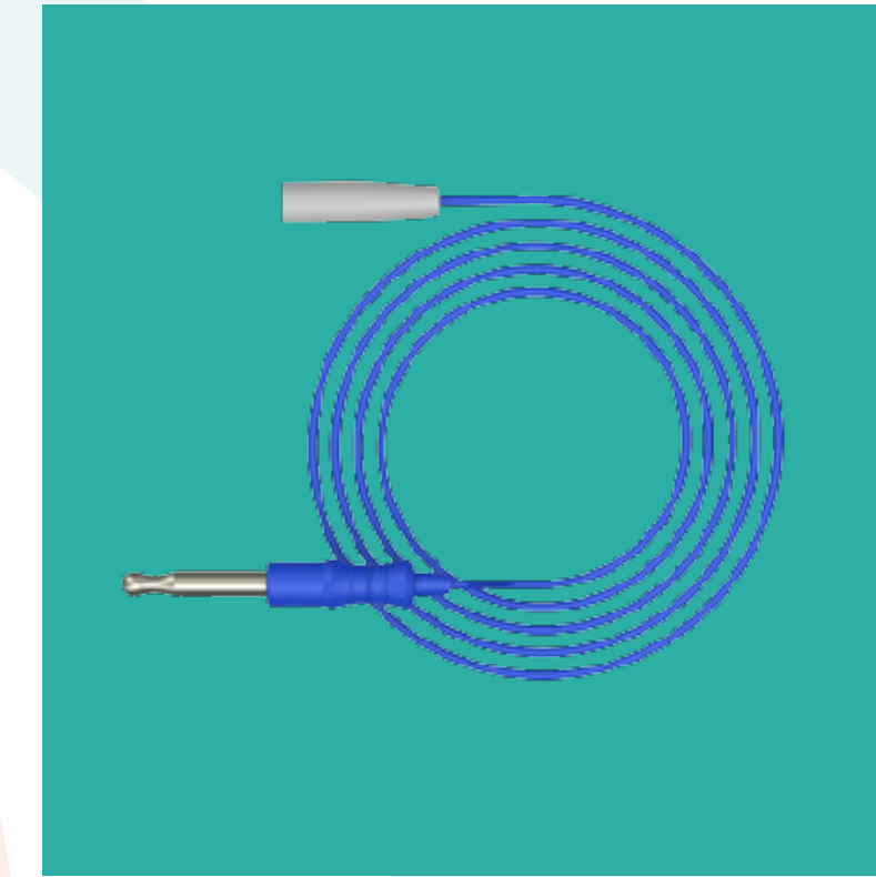
Cabo p/ Pinça Monopolar 3,0m. Conectores: Macho Ø 8mm e Macho Isolado Padrão MF (Pino Cônico Ø D = 2,7 x d = 2,1mm). (MC-09)
