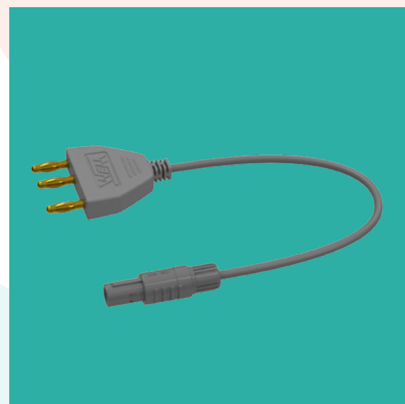
Cabo ESU p/ Bisturi Eletrônico 170mm
