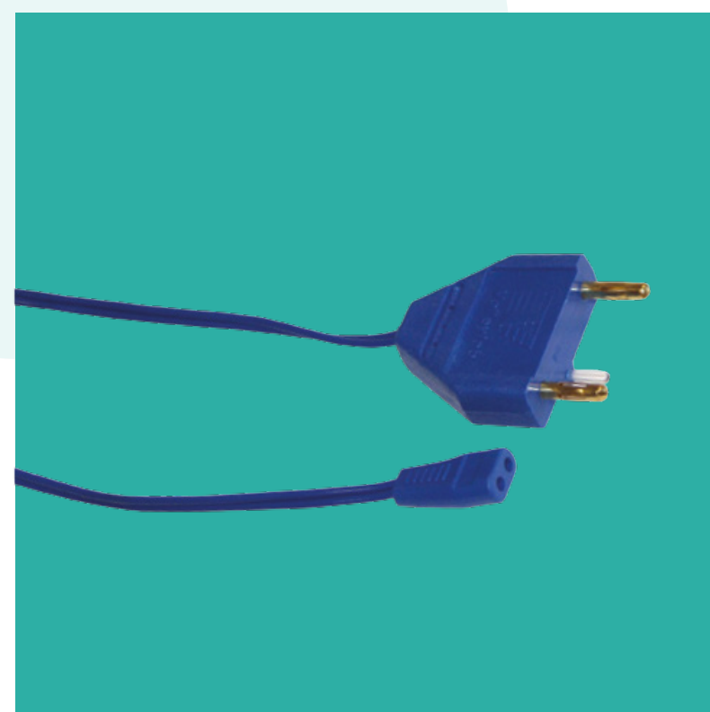
Cabo Pinça Bipolar Valleylab™ Descartável 12' (3,6m) E0512
