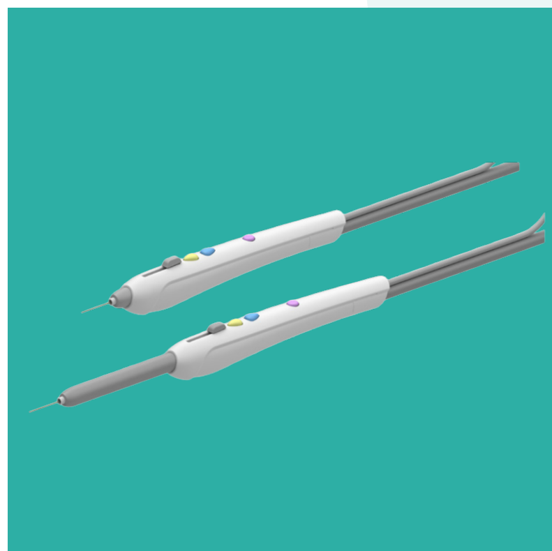
Caneta Eletrocirúrgica Multifuncional Descartável c/ Spinner de 25 mm. Indicada p/ Uso c/ Argon 2 e Argon 4 (Griff) 07994
